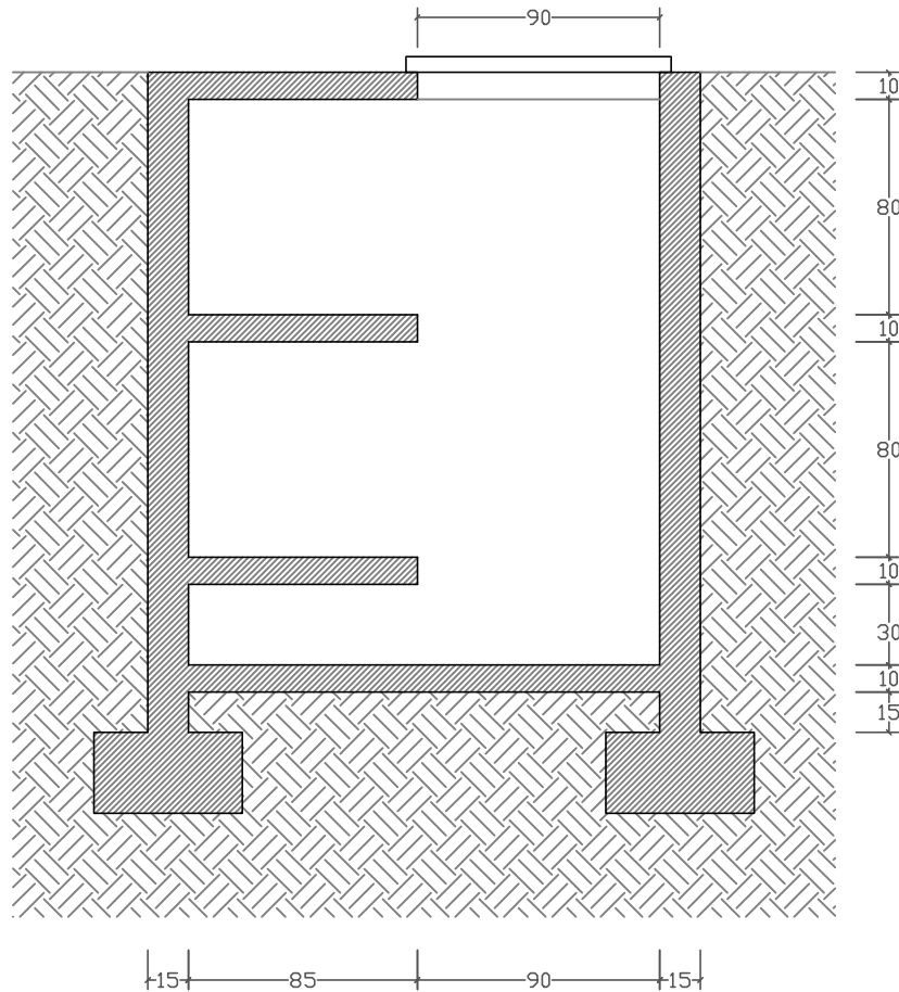
SEZIONE
